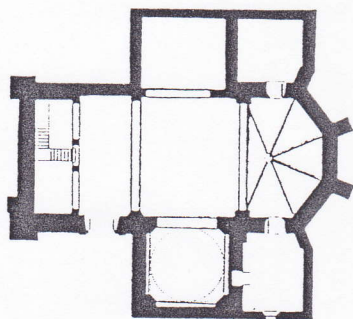
Planta de la Iglesia de Nuestra Señora de las Nieves, gótica, en la que destaca su cabecera poligonal.
